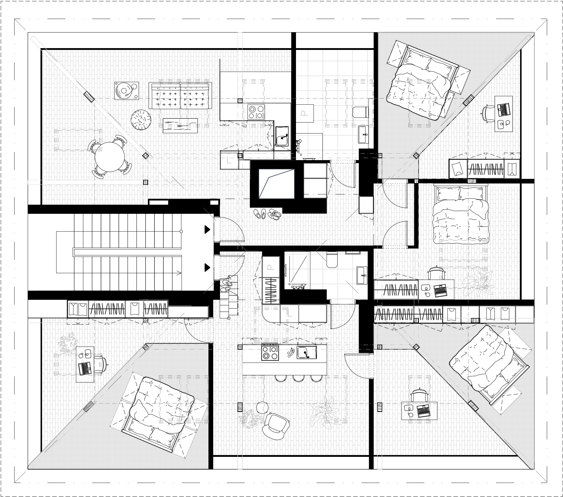
PÔDORYS PODKROVIA
